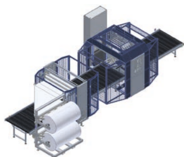
Configuración bobinas laterales Configurações das bobinas laterais
