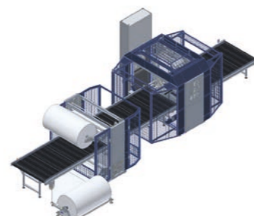
Configuración bobinas arriba y lateral Configurações das bobinas superior e lateral
