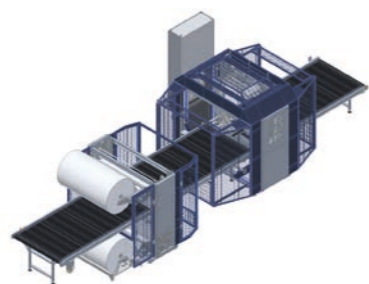
Configuración bobinas arriba y abajo Configurações das bobinas superior e inferior
